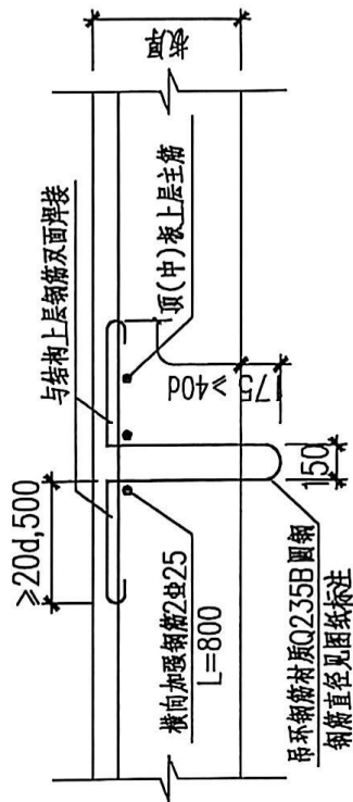
顶板吊环详图
