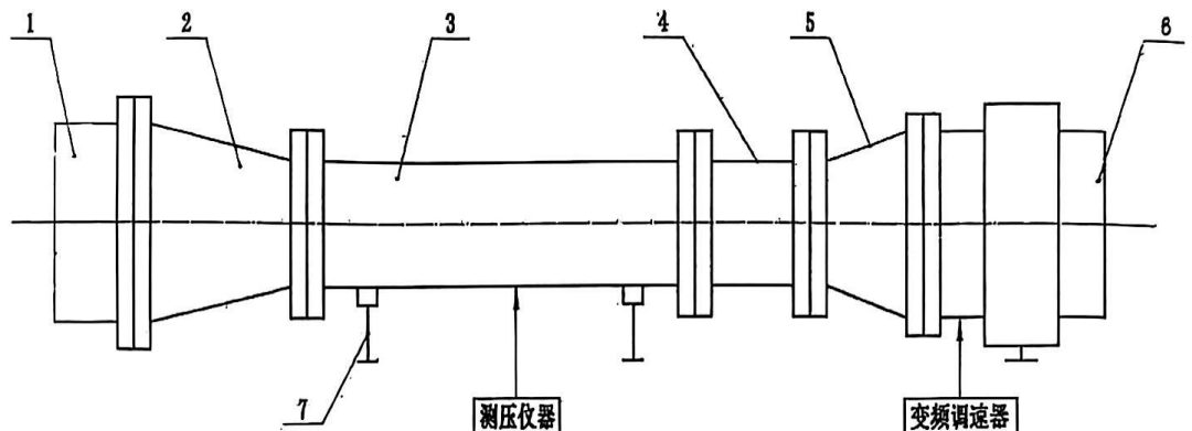
图 G.1 通风性能试验装置示意图
