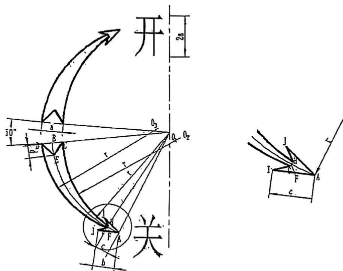
图 6 开关指示箭形标志尺寸示例
