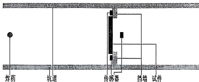
图 A. 3 试验装置示意图 (a-a)
