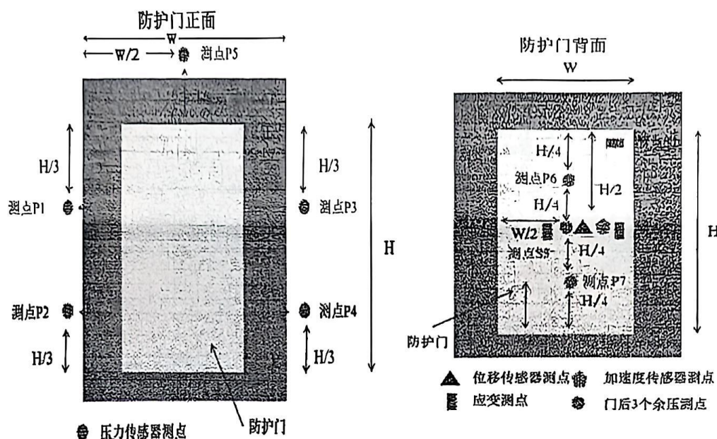
图A.4 传感器布点示意图
