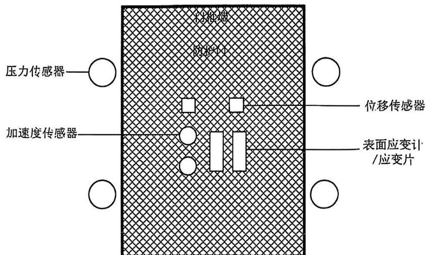
(b) 传感器布置图
