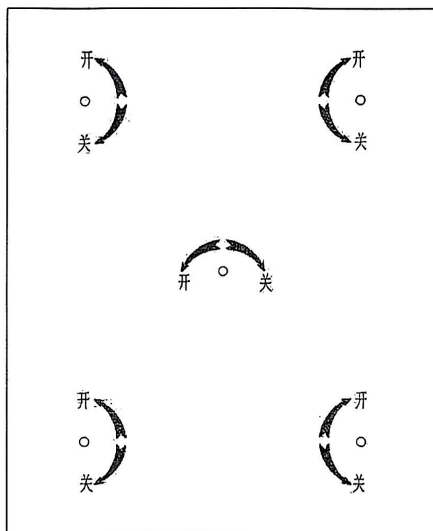
图 5 开关指示箭形标志位置示例
