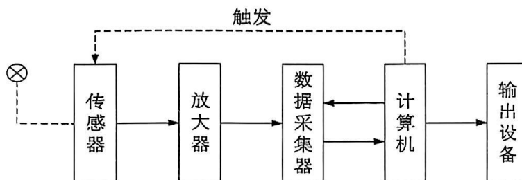
图 A. 1 测试系统工作原理示意图
